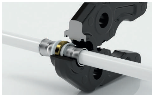
Matriz de prensagem TH
