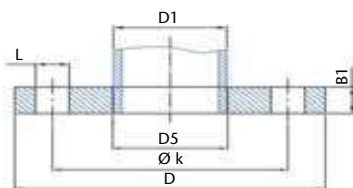
FLANGE PLANA EM ALUMÍNIO BRANCO DIN 2642
